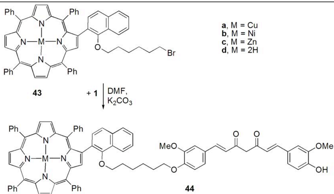
Figura 35. Curcuminoid porfirinas.
